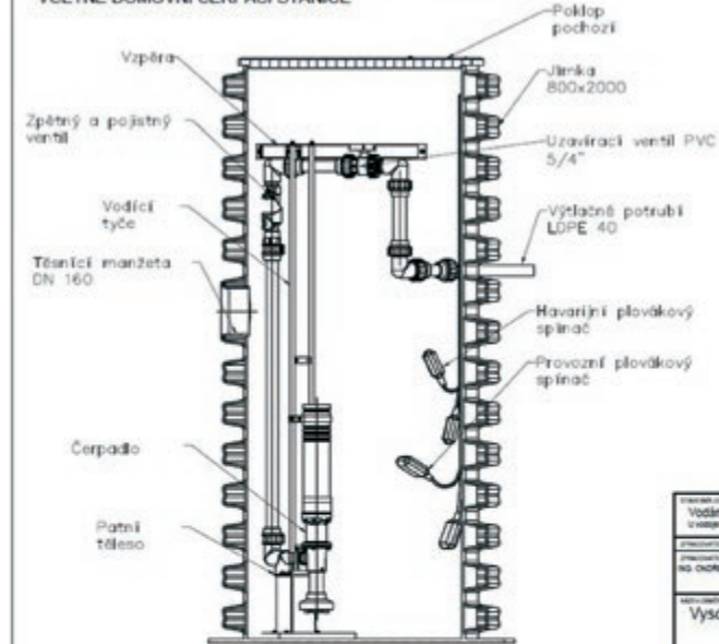
VZOROVÝ PODELNÝ PROFIL TLAKOVÉ KANALIZAČNÍ PŘÍPOJKY VČETNĚ DOMOVNÍ ČERPACÍ STANICE
